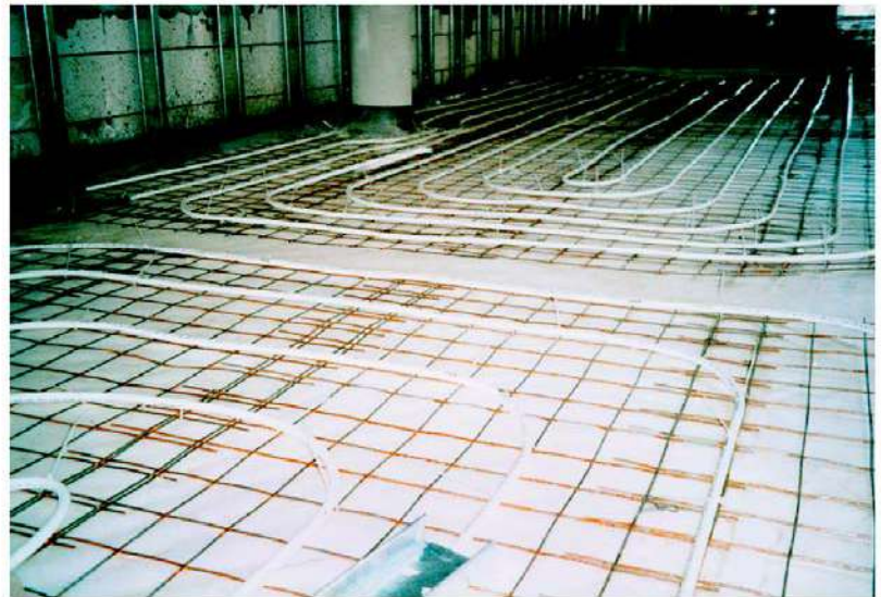
Fig. 12: Sistema de malla soporte de tubos
